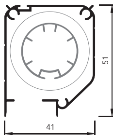
Kassette 4151 Kettenzug
