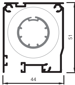
Kassette 4451 Federzug
