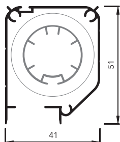
Cassonetto 4151 con catenella
