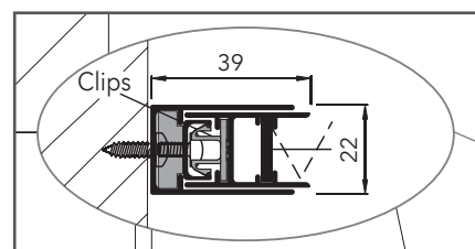
Montaggio in nicchia
