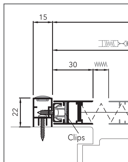
Montaggio frontale
