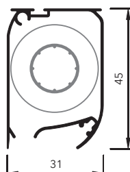
Cassonetto 3145 a molla
