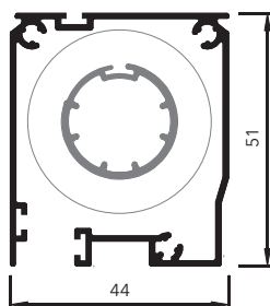
Cassonetto 4451 a molla
